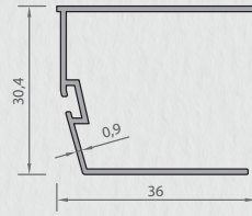
6476 KAPI KARŞILIK PROFİLİ 0,276 kg/mt
