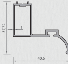
2366 KISA KAPI KARŞILIK PROFİLİ 0,341 kg/mt
