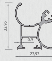
8509 KÖŞE KIRIŞLI DİKME PROFİLİ 0,374 kg/mt
