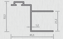
3100 KAPI KARŞILIK PROFİLİ 0,345 kg/mt
