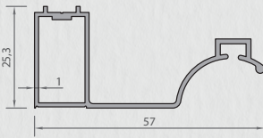
2367 UZUN KAPI KARŞILIK PROFİLİ 0,406 kg/mt
