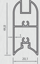
3095 CAM KABİN PROFİLİ 0,519 kg/mt
