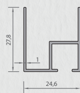
6361 U PROFİLİ 0,266 kg/mt
