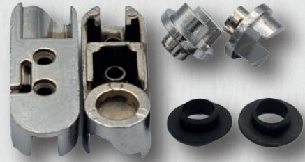
AY-49 SULUKLU BOY MENTEŞE
