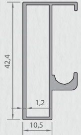
6302 İÇ RAY PROFİLİ 0,415 kg/mt
