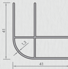
2384 AÇILI BAĞLI DİKME PROFİLİ 0,521 kg/mt
