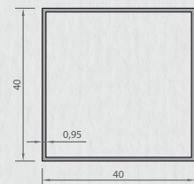
2116 KUTU PROFİLİ 0,403 kg/mt
