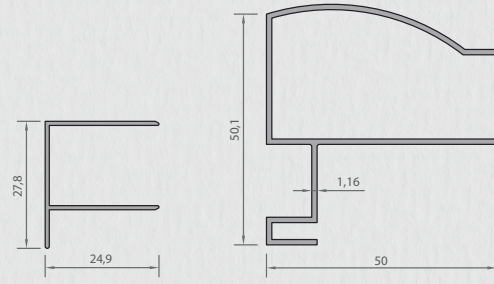
6091 KAPI KARŞILIK PROFİLİ 0,184 kg/mt
