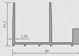
6360 U PROFİLİ 0,553 kg/mt
