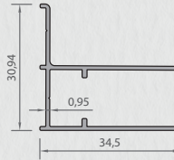
2373 DUVAR DİKMESİ PROFİLİ 0,274 kg/mt
