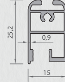
6472 DİKME PROFİLİ 0,309 kg/mt
