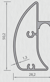
3864 RAY PROFİLİ 0,536 kg/mt
