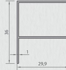
6303 KAPI KARŞILIK PROFİLİ 0,280 kg/mt
