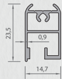
6473 DİKME PROFİLİ 0,249 kg/mt
