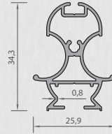
8508 ORTA DİKME PROFİLİ 0,374 kg/mt
