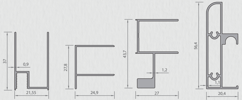
6090 CAM PROFİLİ 0,265 kg/mt
