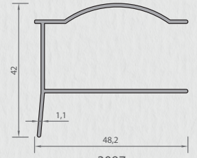
3097 KAPI KARŞILIK PROFİLİ 0,390 kg/mt
