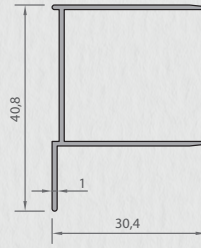
6475 KAPI KARŞILIK PROFİLİ 0,250 kg/mt
