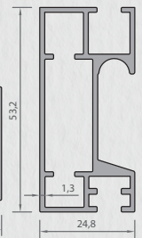
9051 RAY PROFILI 0,750 kg/mt
