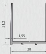
6359 U PROFİLİ 0,317 kg/mt
