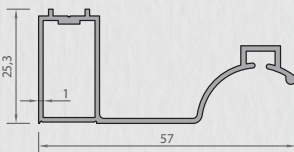
2367 LONG DOOR STRIKE PROFILE 0,406 kg/mt
