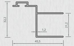
3100 DOOR STRIKE PROFILE 0,345 kg/mt
