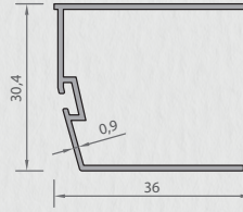
6476 DOOR STRIKE PROFILE 0,276 kg/mt
