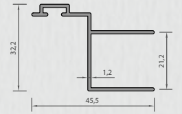
3100 ملف تعريف خربة الباب كجم / طن متري 0,345
