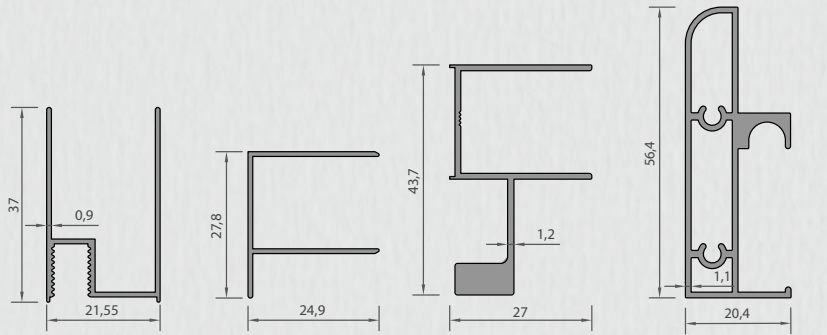
6090 ملف تعريف الزجاج كجم / طن متري 0,265
