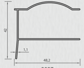
3097 ملف تعريف خربة الباب كجم / طن متري 0,390
