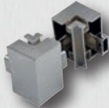
إسفين الزاوية (السكة) - AY 306 (2 قطعة)
